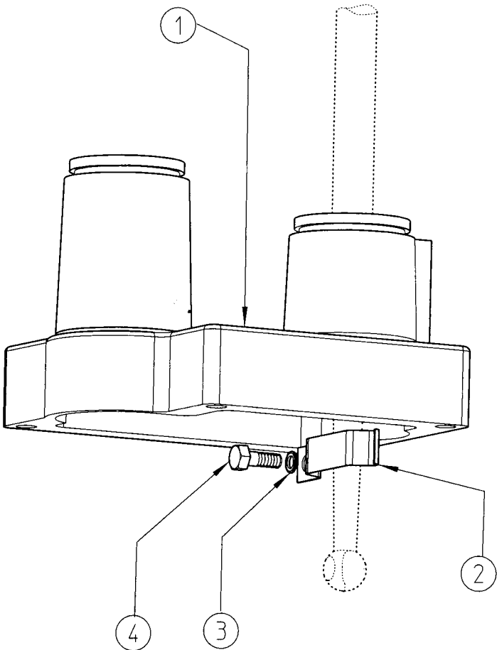
v.tapa.desconector
